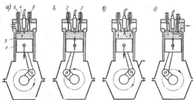
Рисунок 1 - Рабочий процесс четырехтактного двигателя
