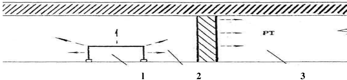
Рис. 3.1. Звукоизолирующее ограждение: 1 - источник шума; 2 - шумное помещение; 3 - изолируемое помещение; РТ - расчетная точка
