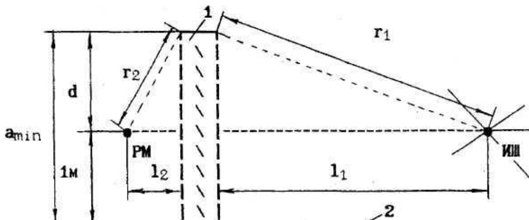
Рис. 3.4. Акустическое экранирование:
